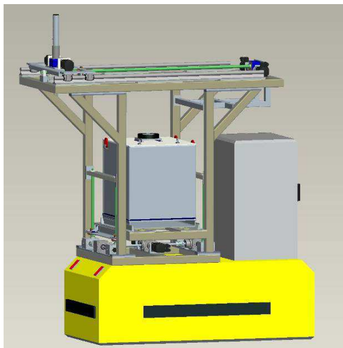
Fig 3: Dispositivo di movimentazione del target
