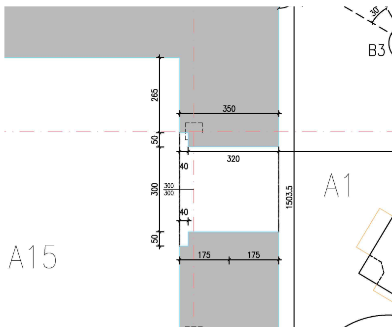
Fig 5. Particolare porta A15/A1
