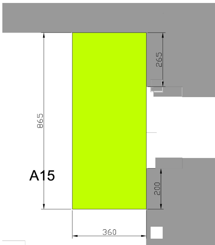
Fig 6. Particolare riservazione a pavimento porta 4
