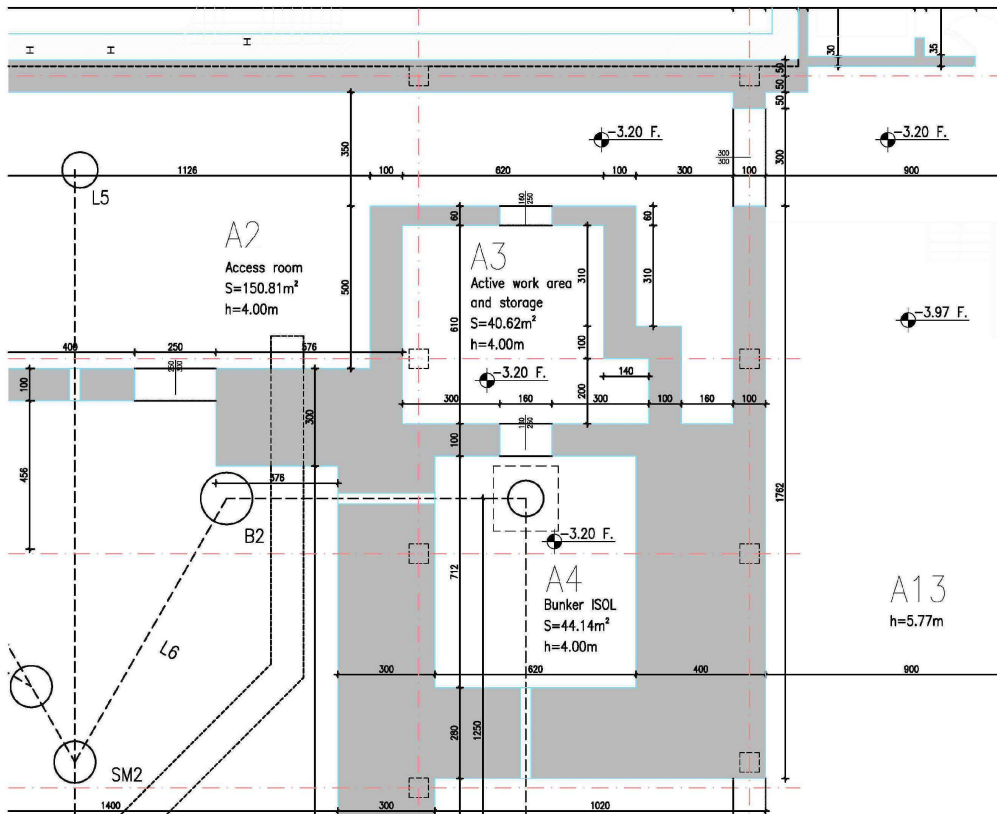
Fig 6. Particolare pianta interrato locali A, A3, A2
