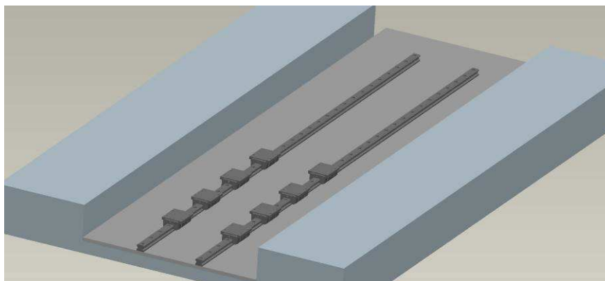
Fig 1: Sistema di guida a ricircolazione di sfere inserito nella fossa prospiciente la soglia
